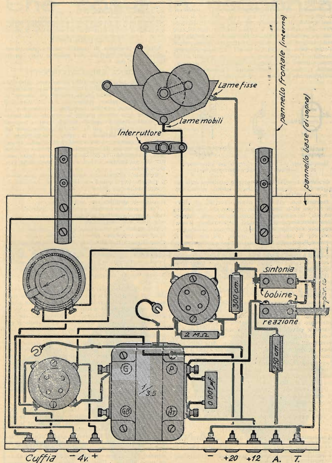
Schema costruttivo del « Bigrivox ».
